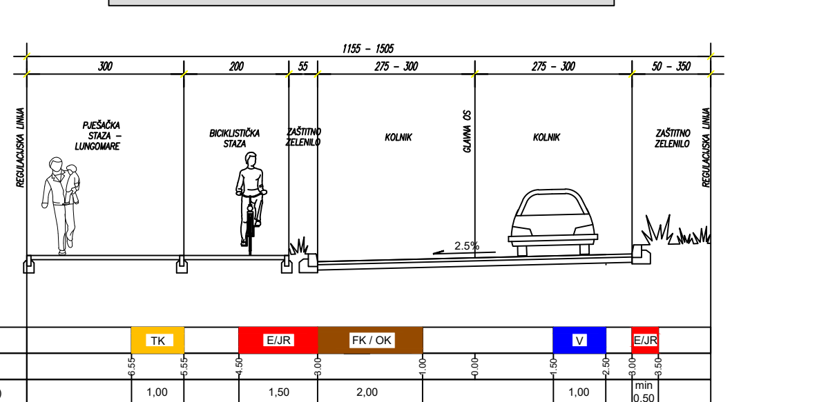
OSTALA ULICA - NAČELNI POPREČNI PRESJEK A4
