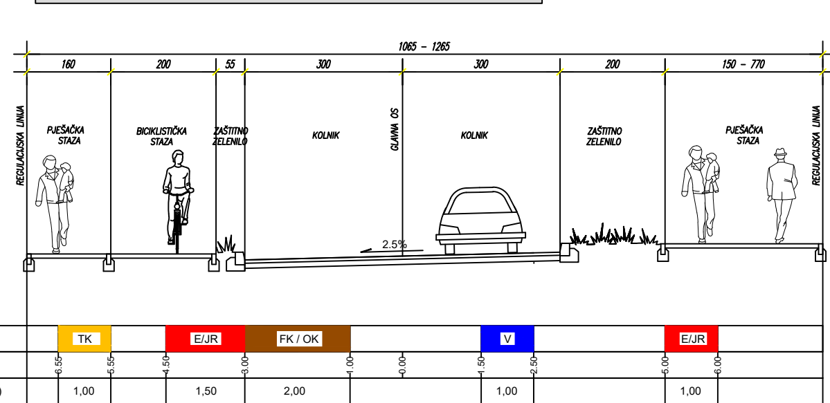
PRIMORSKA ULICA - NAČELNI POPREČNI PRESJEK A2
