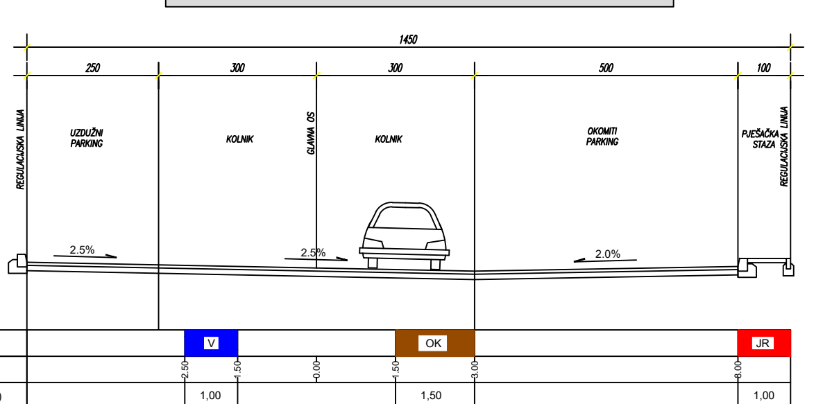
ULICA PLASICA - NAČELNI POPREČNI PRESJEK A5
