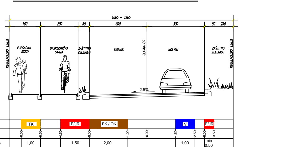
PRIMORSKA ULICA - NAČELNI POPREČNI PRESJEK A3
