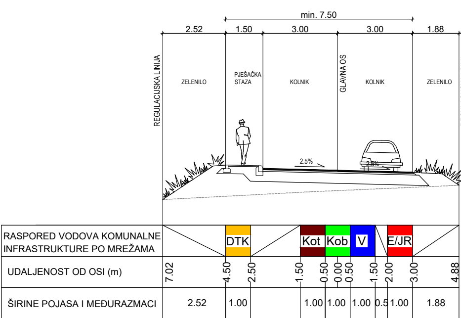
PRESJEK B5-B5
