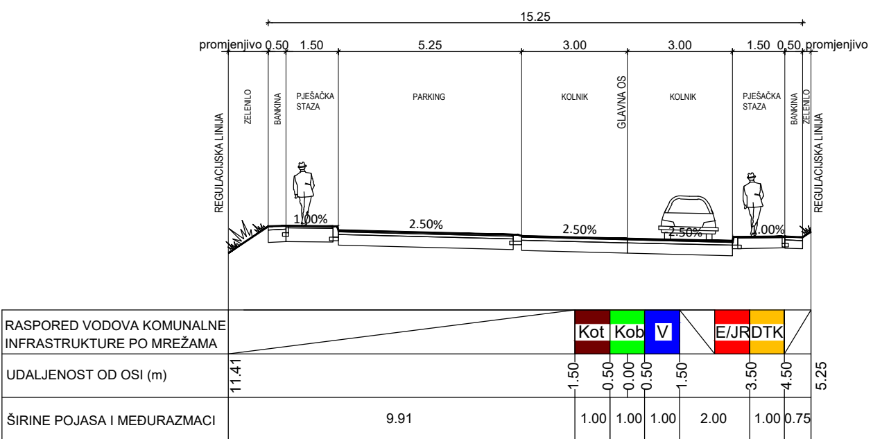
PRESJEK B4-B4
