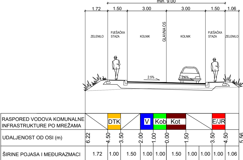
PRESJEK B1-B1
