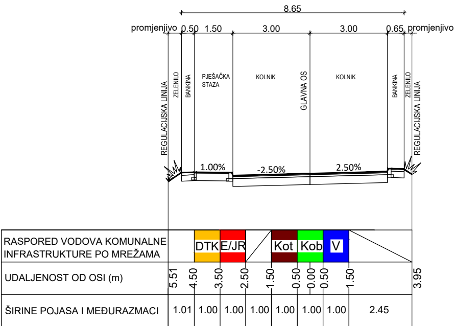
PRESJEK B2-B2
