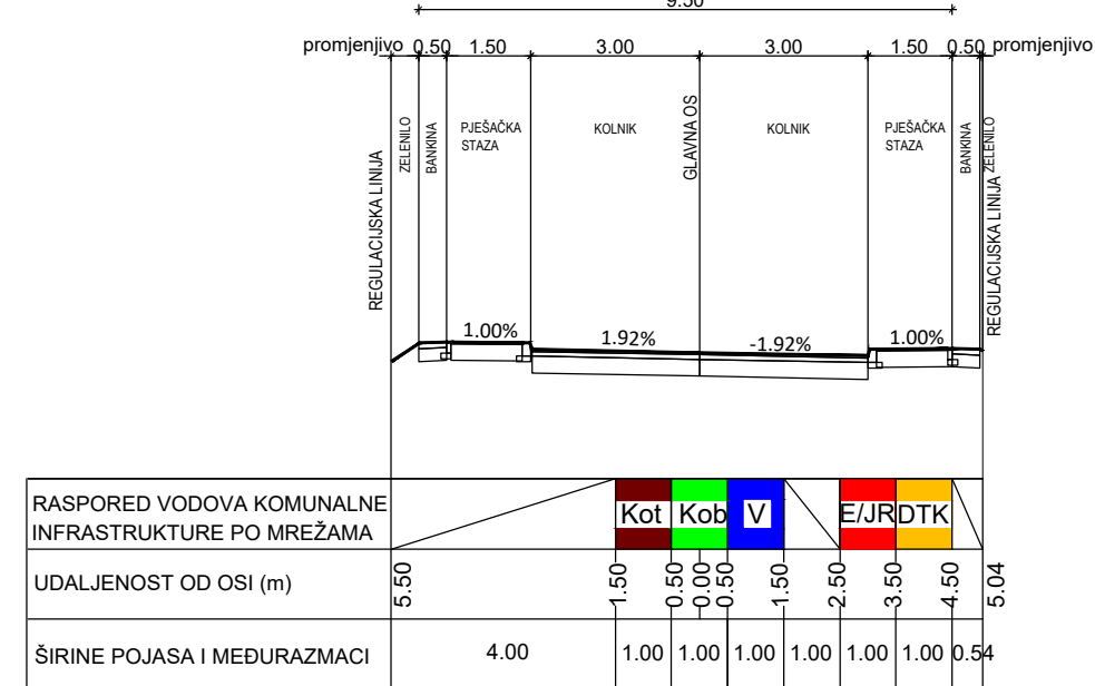
PRESJEK B5-B5
