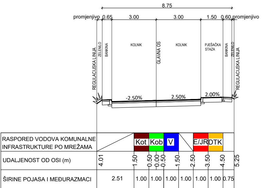
PRESJEK B2-B2
