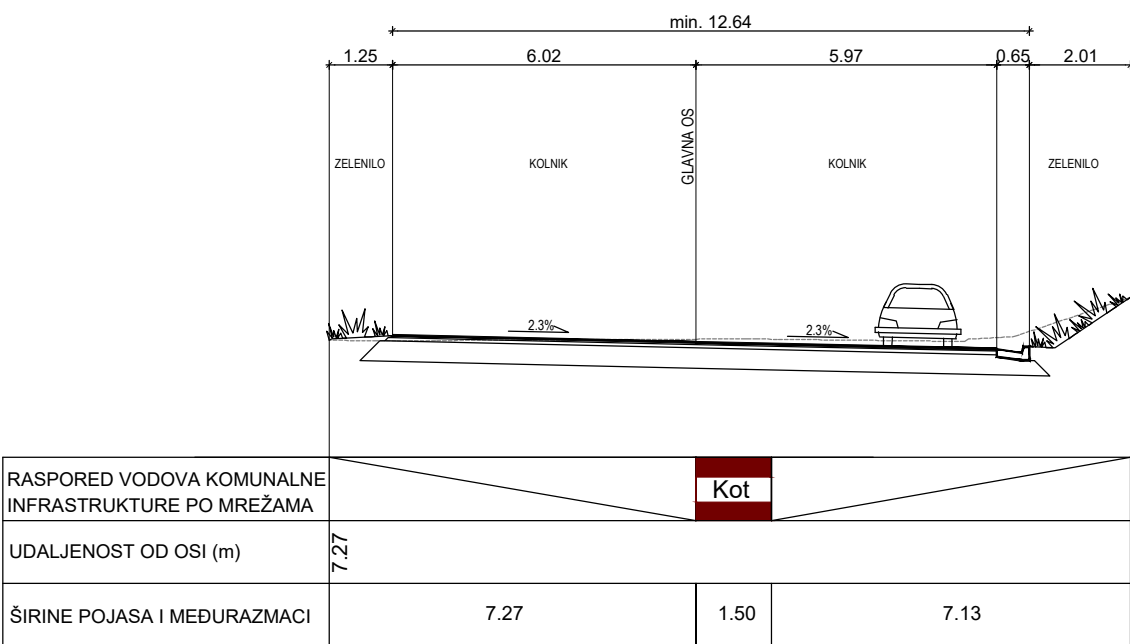
PRESJEK A2-A2
